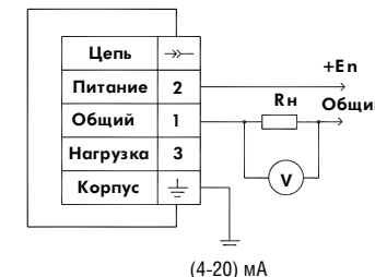
Схема внешних соединений
