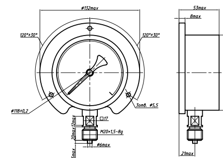
Вариант исполнения с электрической подсветкой циферблата
